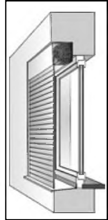
комбинированный монтаж коробом внутрь
